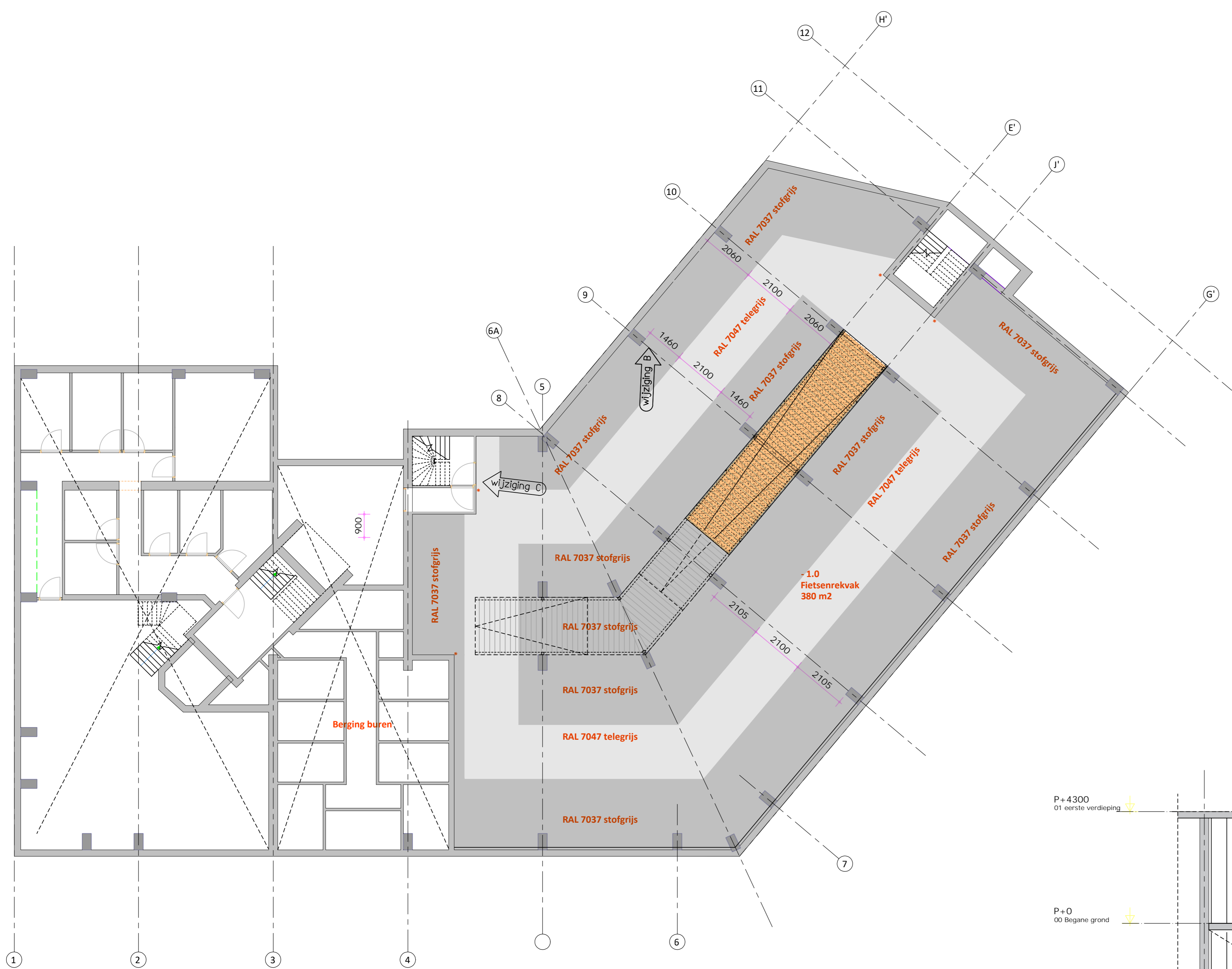
Kelder 1:100
