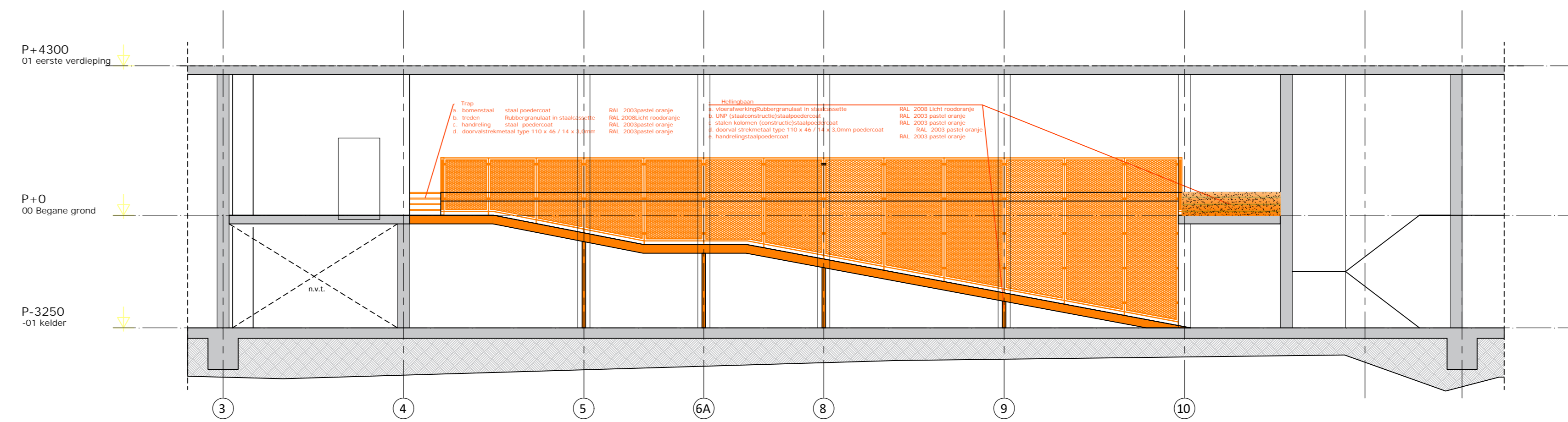
Langsdoorsnede hellingbaan 1:100
