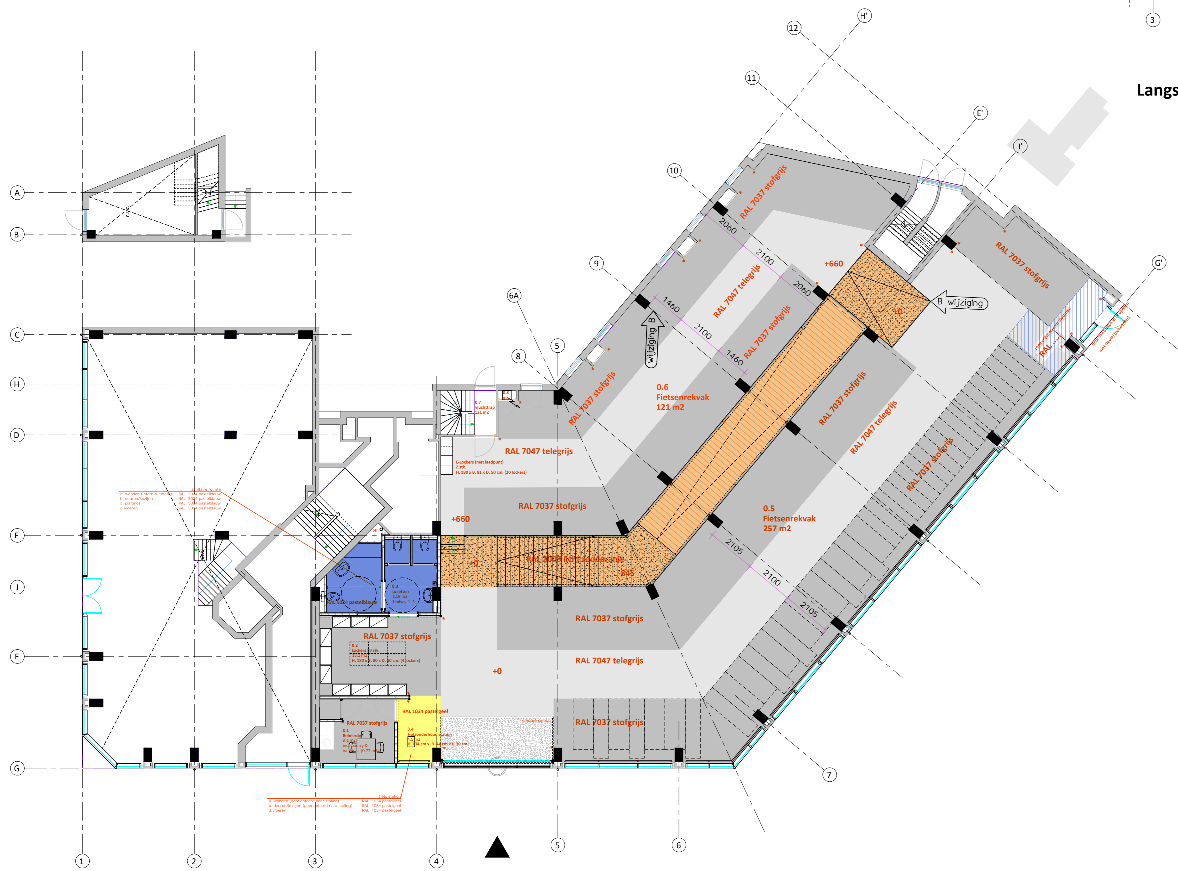
Begane grond 1:100
